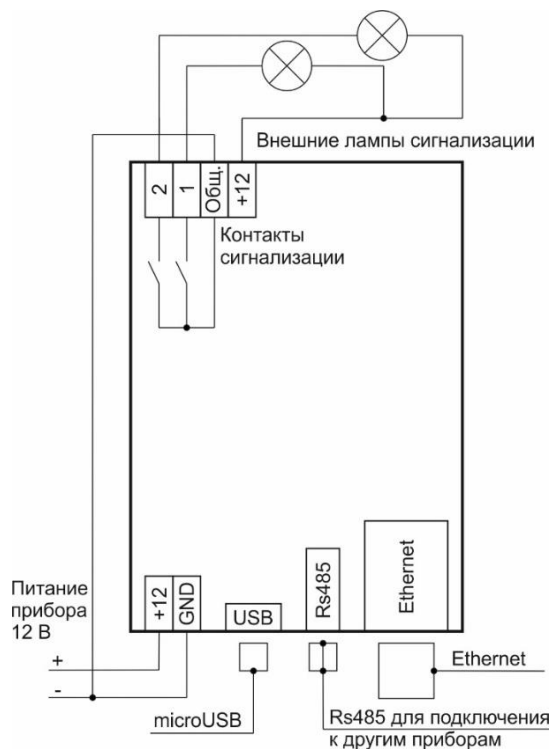
Рисунок 1а – Схема подключения сигнализации
