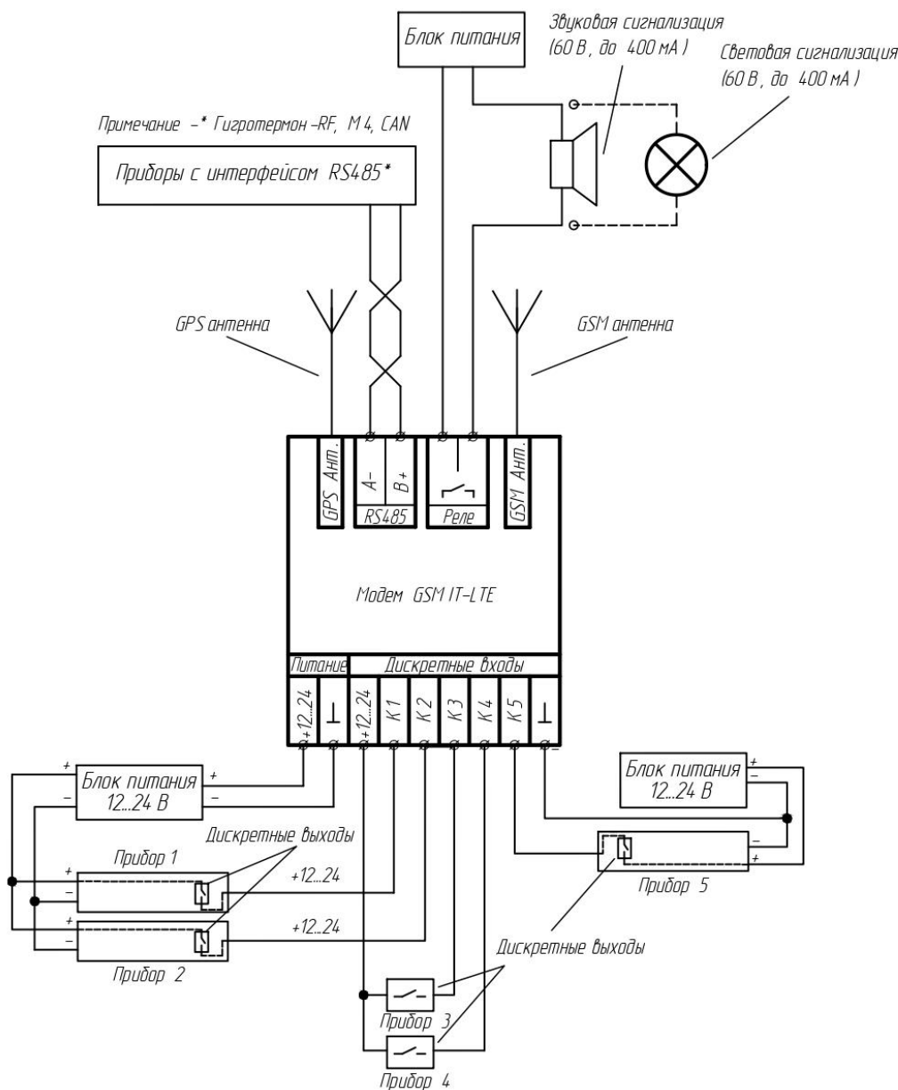
Рисунок 2 – Схема подключения внешних устройств
