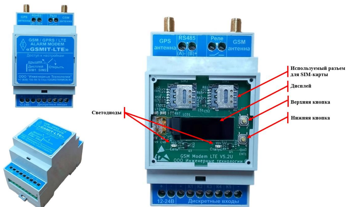
Рисунок 1 – Общий вид устройства
